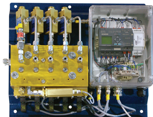
Auto Cascade
